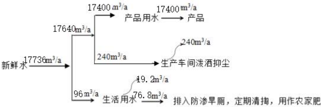
图 3-1 水平衡图
